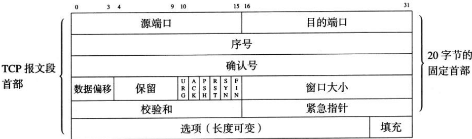
(b) TCP 段头结构
